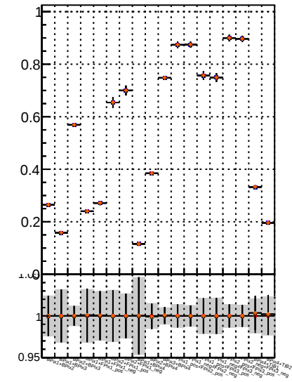
Fake rate vs. BGM noMS BGM noMS PL BGM noMS PL MS BGM noMS PL MS mod MS
