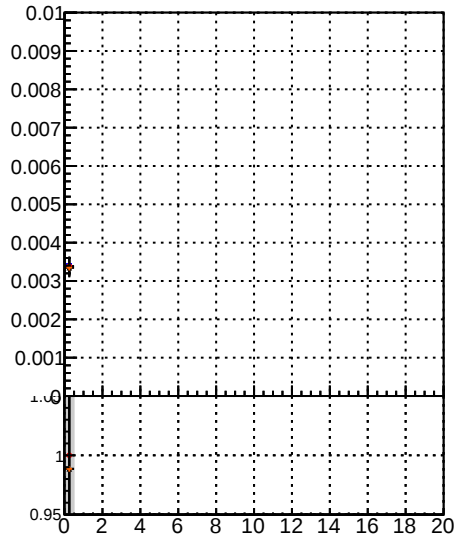
Fake rate vs. BGM noMS BGM noMS PL BGM noMS PL MS BGM noMS PL MS mod MS
