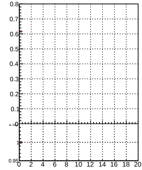
Fake rate vs. BGM noMS BGM noMS PL BGM noMS PL MS BGM noMS PL MS mod MS
