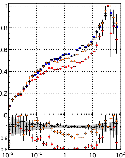
DOM noMS DOM MS PL orig/DOM orig MS pixelLessOrig/DOM mod MS
