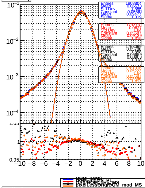
pull of \phi parameter
