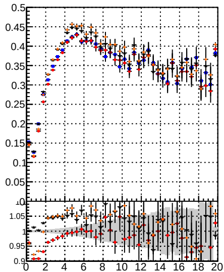
Fake rate vs. BGM pBMS BGM+PLMS PixelLessOrBGM mod MS
