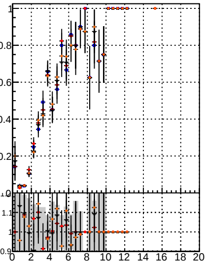
Fake rate vs. BQM noMS BQM noMS PL BQM noMS PL MS BQM noMS PL MS mod MS
