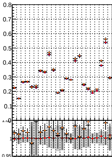
Fake rate vs. — BGM noMS — BGM noMS PLMS — BGM noMS PLMS mod MS — BGM noMS PLMS mod MS
