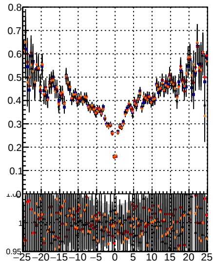
Fake rate vs d —●— BGM noMS —●— BGM noMS PLMS —●— pixelLess on BGM mod MS
