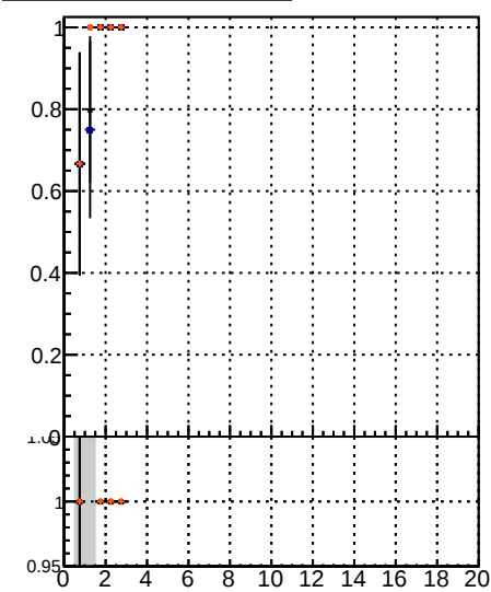
Fake rate vs. BQM, noMS BQM, noMS, PL BQM, noMS, PL, LMS PixelLessOrandom mod MS
