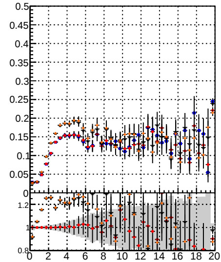
Fake rate vs. BGM noMS BGM noMS PLMS BGM noMS PLMS mod MS BGM noMS PLMS mod MS
