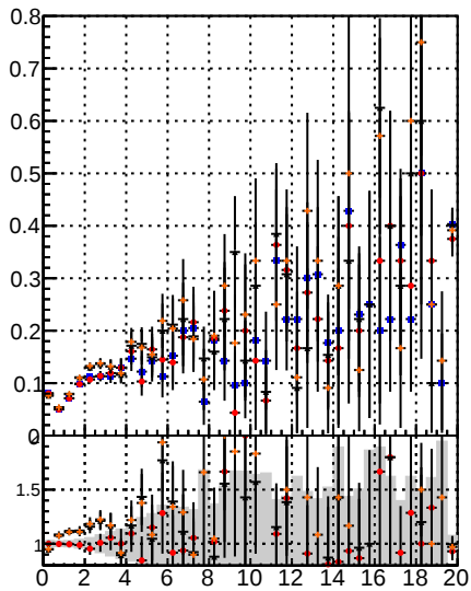
Fake rate vs. BGM noMS BGM noMS PLMS BGM noMS PLMS mod MS BGM noMS PLMS mod MS
