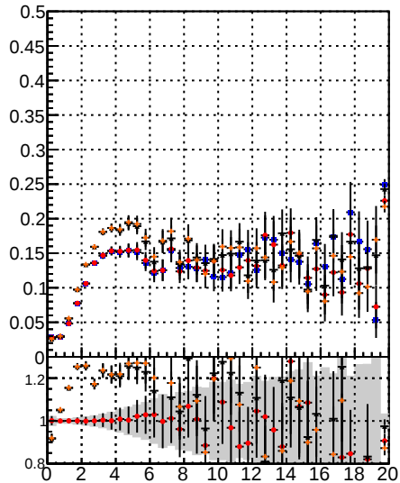
Fake rate vs. BGM noMS BGM noMS PLMS PixelLess or BGM mod MS
