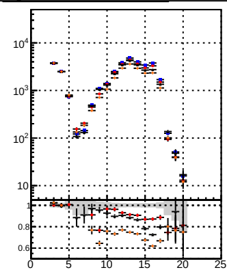
N of reco track vs hit DOM noMS DOM modMS DOM noMS PL DOM modMS PL origDOM pixelLess OrigDOM DOM mod MS
