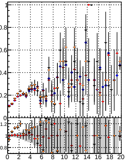
Fake rate vs. BQM noMS BQM+noMS PLMS BQM+PLMS mod MS
