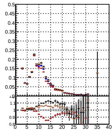
Legend: DQM_noMS DQM_moMS_PL Orig/DQM_orig_MS pixelLessOrig/DQM_mod_MS
