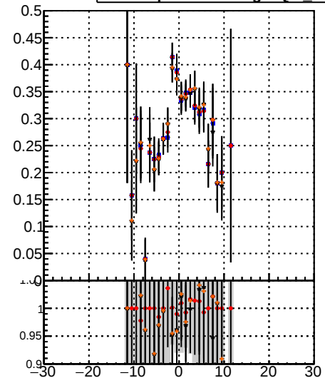
Fake rate vs v DOM noMS DOM noMS PL Orig/DOM orig MS pixelLessOrig/DOM mod MS
