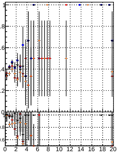
Fake rate vs. BQM noMS BQM noMS PL BQM noMS LMS PixelLessOrandom mod MS
