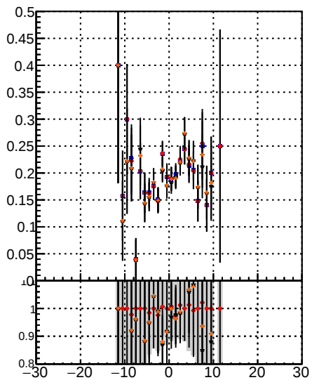
Fake rate vs d BQM noMS BQM noMS PL pixelLess noMS BQM mod MS
