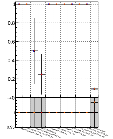
Fake rate vs. BQM, noMS BQM, noMS, PL PixelLessOrandom mod MS
