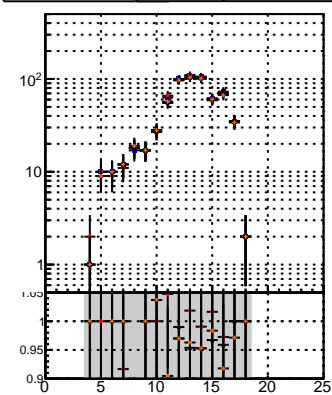
N of reco track vs hit DQM_noMS DQM_noMS_PL orig/DQM pixelLessOrig/DQM DQM_mod MS
