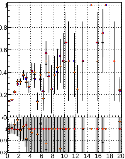
Fake rate vs. BQM noMS BQM noMS PLMS PixelLessOrandom BQM mod MS
