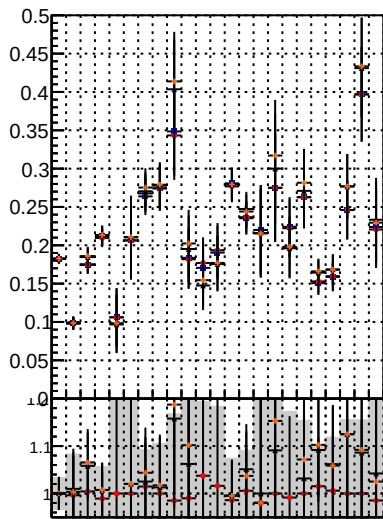
Fake rate vs. BQM noMS BQM noMS PLMS PixelLessOrandom BQM mod MS
