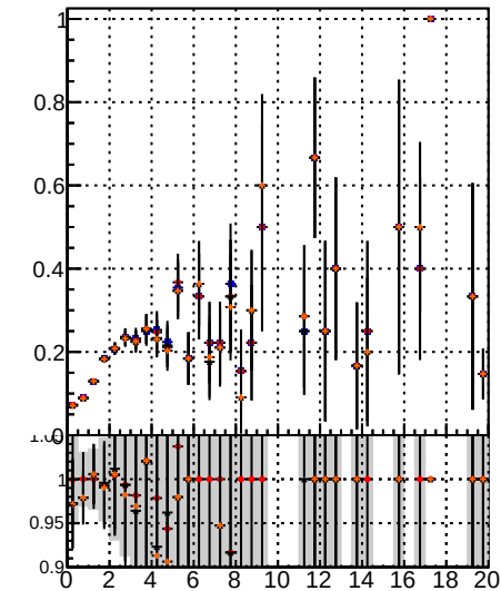
Fake rate vs. BQM noMS BQM noMS PLMS BQM noMS PLMS mod MS PixelLessOrNoBQM
