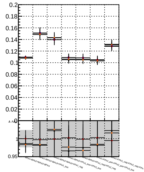
Fake rate vs. BQM noMS BQM noMS PLMS BQM noMS PLMS mod MS PixelLessOrNoBQM
