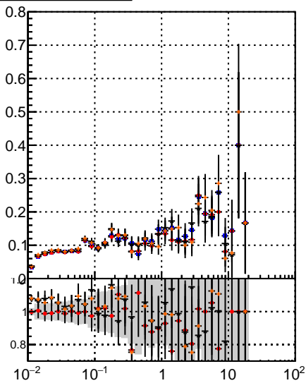
Fake rate vs v —■— DQM_noMS —●— DQM_noMS_PL —▲— Orig/DQM_orig_MS —▼— pixelLessOrig/DQM_mod_MS
