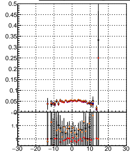
Fake rate vs v —■— DQM_noMS —●— DQM_noMS_PL —▲— Orig/DQM_orig_MS —▼— pixelLessOrig/DQM_mod_MS
