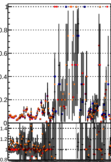
Fake rate vs. BQM, noMS BQM, noMS, PLMS pixelLess or random MS mod MS
