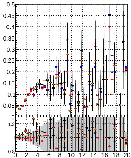
Fake rate vs. BQM, noMS BQM, noMS, PLMS pixelLess or random MS mod MS
