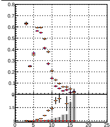
—●— DQM_noMS —●— DQM_noMS_PL —●— Orig/DQM_orig_MS —●— pixelLessOrig/DQM_mod_MS
