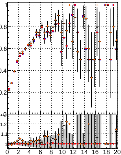
Fake rate vs. DGM noMS DGM noMS PLMS DGM noMS PLMS mod MS PixelLessDGM
