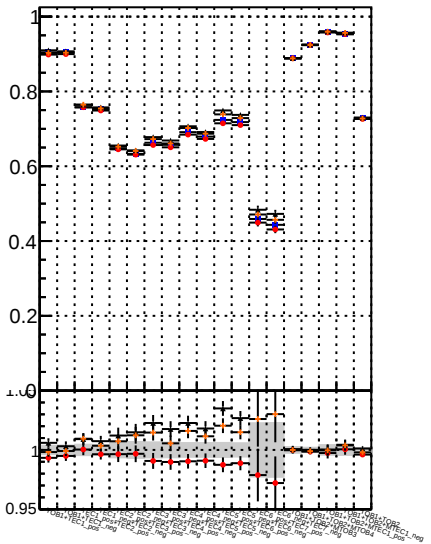
Fake rate vs. BQM noMS BQM noMS + PL OLS noMS + PL pixelLess or BQM mod MS
