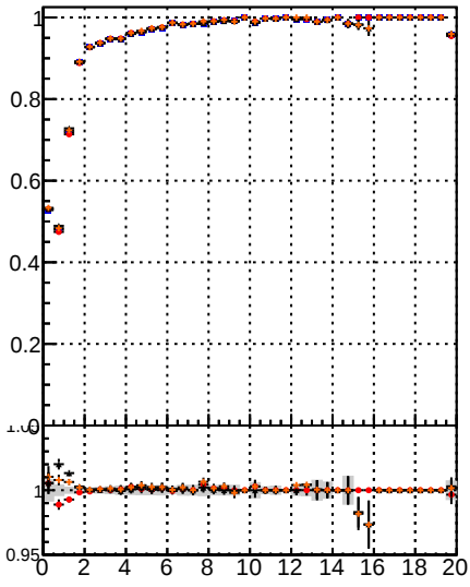
Fake rate vs. BQM noMS BQM noMS + PL OLS noMS + PL pixelLess or BQM mod MS
