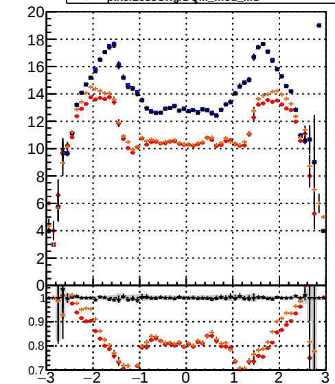
mean hit — DQM_noMS — DQM_moMS_PL — Orig/DQM_orig_MS — pixelLessOrig/DQM_mod_MS
