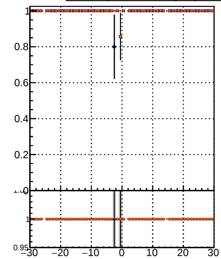
Fake rate vs vertpos DOM-noMS DOM-trimMS-PL Orig/DOM-orig-MS pixelLessOrig/DOM mod MS
