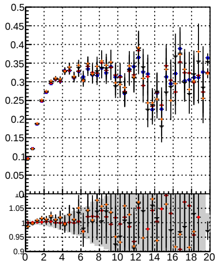
Fake rate vs. BQM, DQM, PLMS, DQM mod MS
