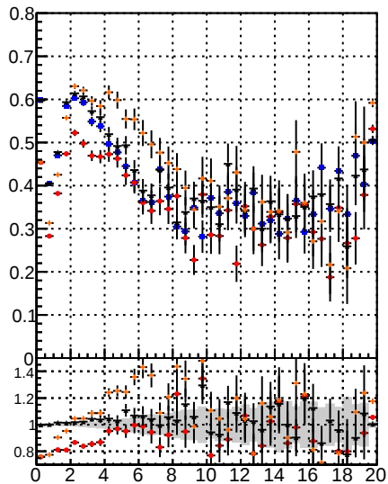
Fake rate vs. BQM noMS BQM noMS PLMS PixelLess or BQM mod MS
