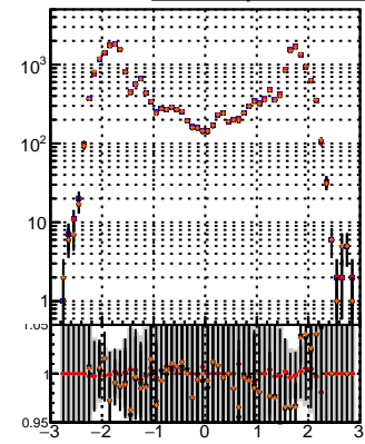
N of reco track vs \eta BQM DQM MS PLMS orig/pixelLessOrig pixelLessOrig DQM mod MS
