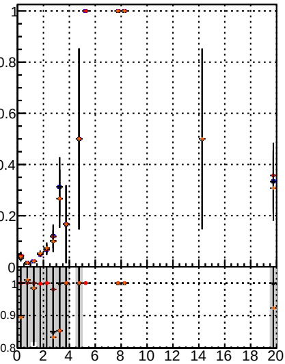
Fake rate vs. BOM noMS BOM noMS PL BOM noMS PL MS BOM noMS PL MS mod MS
