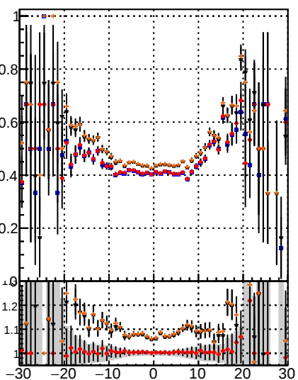
Fake rate vs d DQM noMS DQM noMS PLMS pixelLessOrandom mod MS
