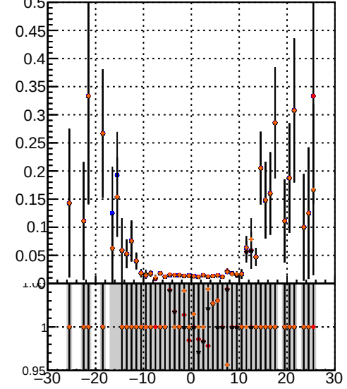
Legend for all plots: —●— DQM TT MS —●— DQM TT MS detT —●— DQM TT MS detT1 —●— DQM TT MS detT09 Efficiency vs sim PV z
