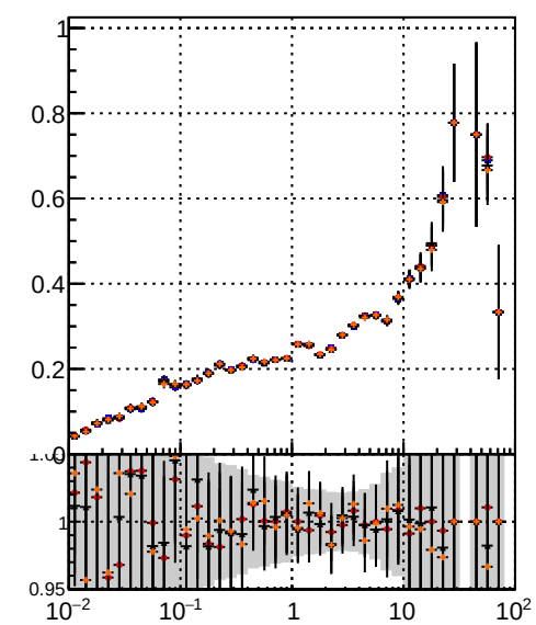
Legend for all plots: —●— DQM TT MS —●— DQM TT MS detT —●— DQM TT MS detT1 —●— DQM TT MS detT09 Efficiency vs sim PV z
