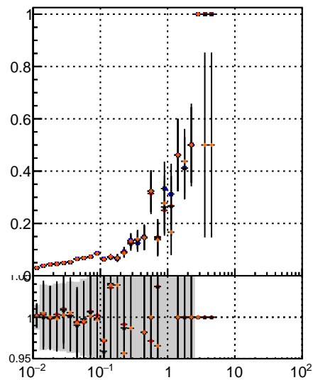
Fake rate vs \sqrt{s} —●— DQM TT MS detT —●— DQM TT MS detT1 —●— DQM TT MS detT09
