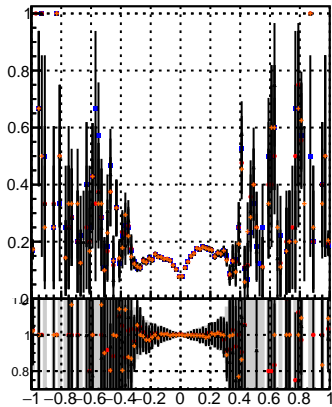
—●— DQM TT MS —●— DQM TT MS detT —●— DQM TT MS detT1 —●— DQM TT MS detT09
