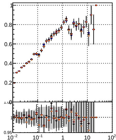
Fake rate vs \sqrt{s} DQM TT MS detT DQM TT MS detT1 DQM TT MS detT109
