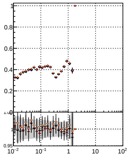
Fake rate vs v DOM TT MS detT detT1 detT109 — — — — — — — — — — — — — — — — — —
