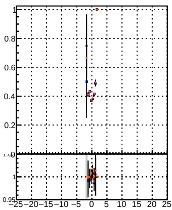
— DOM TT MS — DOM TT MS detT1 — DOM TT MS detT109 — DOM TT MS detT09
