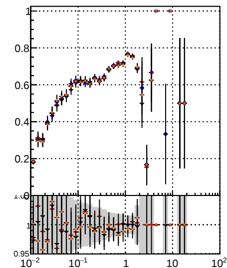
Fake rate vs \sqrt{s} DQM TT MS detT DQM TT MS detT1 DQM TT MS detT09 DQM TT MS detT109
