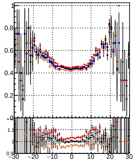
Fake rate vs \nu DQM TT MS detT DQM TT MS detT1 DQM TT MS detT09
