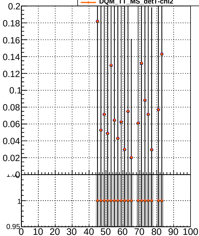
DQM TT MS DQM TT MS detT DQM TT MS detT-dpdq DQM TT MS detT-chi2
