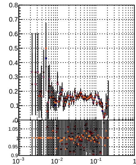
Fake rate vs \overline{b\overline{b}} t\overline{t} MS detT dpdq ch2
