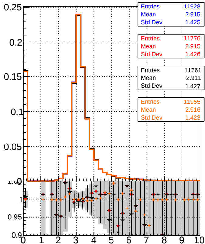
dE/dx estimator 1
