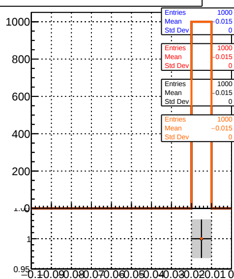
GeneratedTT_MS
