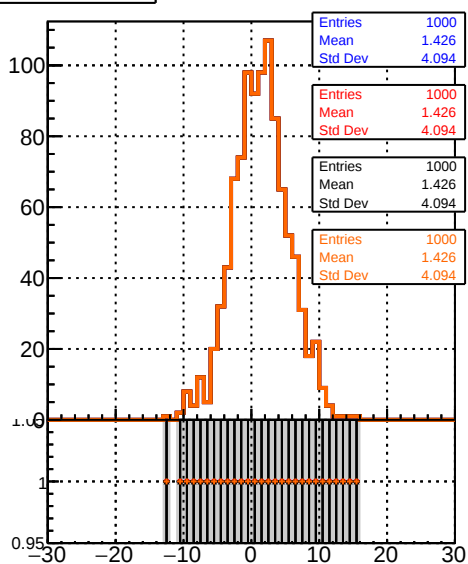
GeneratedPV_Z
