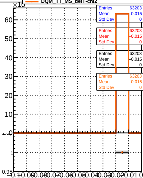
GeneratedTT_MS
