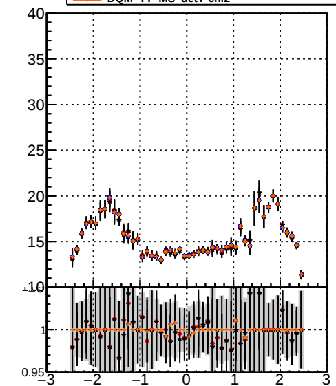
mean hit DQM_TT_MS DQM_TT_MS_detT DQM_TT_MS_detT-dpdq DQM_TT_MS_detT-chi2
