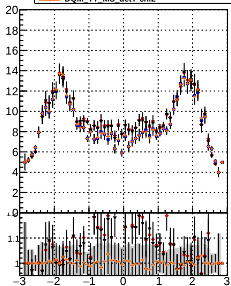
mean hit DQM_TT_MS DQM_TT_MS_detT DQM_TT_MS_detT-dpdq DQM_TT_MS_detT-chi2
