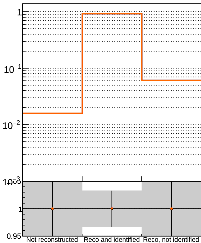
DQM_TT_MS DQM_TT_MS_detT DQM_TT_MS_detT-dpdq DQM_TT_MS_detT-chi2
