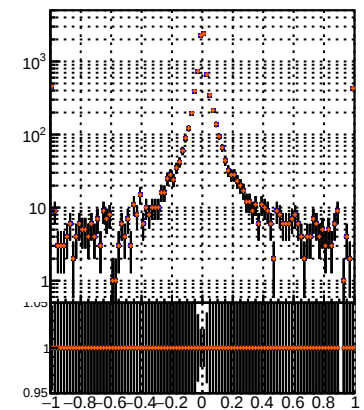
N of sim Legend: DQM_TT_MS DQM_TT_MS_detT DQM_TT_MS_detT-dpdq DQM_TT_MS_detT-chi2
