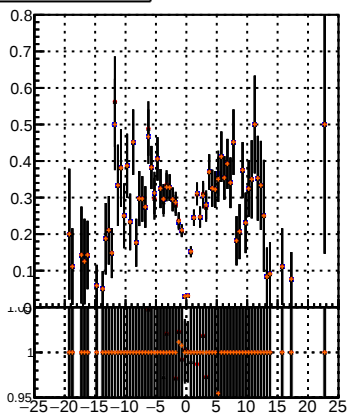
Efficiency Legend: DQM_TT_MS DQM_TT_MS_detT DQM_TT_MS_detT-dpdq DQM_TT_MS_detT-chi2
